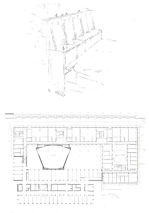
Skizze des Hangsicherungstragwerks (oben) und Grundriss 2. OG, Mst. 1:2000. Der geschützte Hörsaal (Mitte) wird vom GLC-Gebäude und vom Bestand eingefasst. Die Segmentbögen des Hangsicherungstragwerks sind klar zu erkennen.
